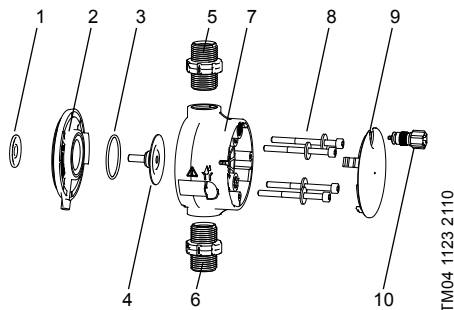
Abb. 40 Membrane und Ventile austauschen
