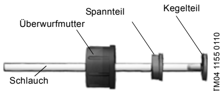
Abb. 8 Hydraulischer Anschluss
