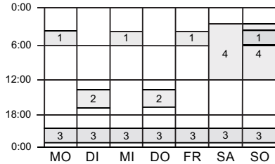
Abb. 28 Wochentimer-Dosierung
