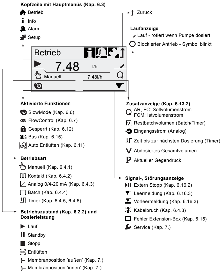
Abb. 14 Übersicht Displaysymbole
