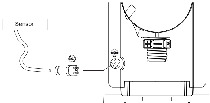
Abb. 11 FlowControl Anschluss
