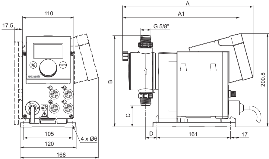
Abb. 4 Maßzeichnung
