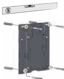
Abb. 5 Montageplatte anbringen
