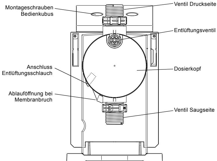
Abb. 3 Rückansicht der Pumpe
