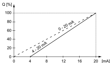
Abb. 16 Analogprofil
