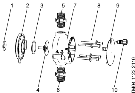
Abb. 23 Membrane und Ventile austauschen
