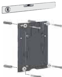
Abb. 5 Montageplatte anbringen
