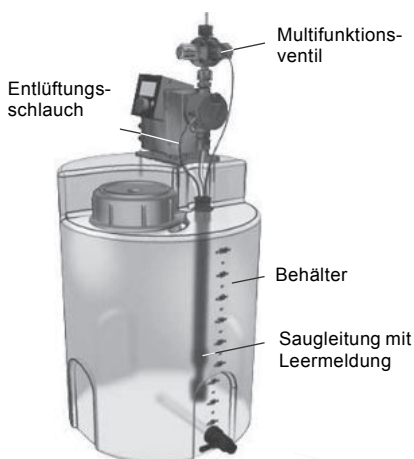
Abb. 9 Installationsbeispiel
