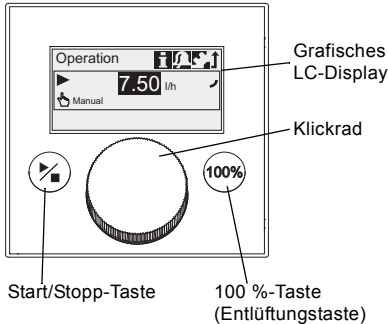
Abb. 12 Bedienfeld
