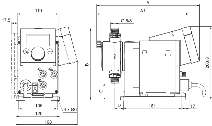
Abb. 4 Maßzeichnung
