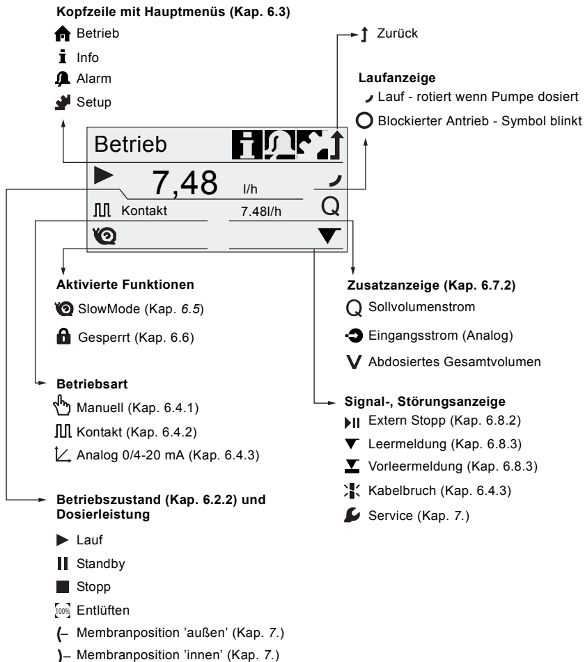
Abb. 13 Übersicht Displaysymbole
